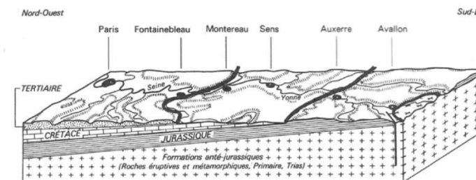
Bloc diagramme schématique du Bassin parisien entre Paris et Avallon (document BRGM)
