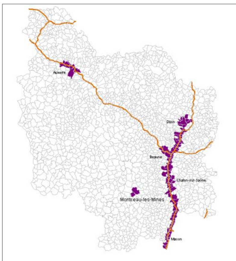
Carte des zones sensibles pour la qualité de l'air
