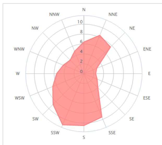
Direction des vents (moyennes de 2009-2015)
